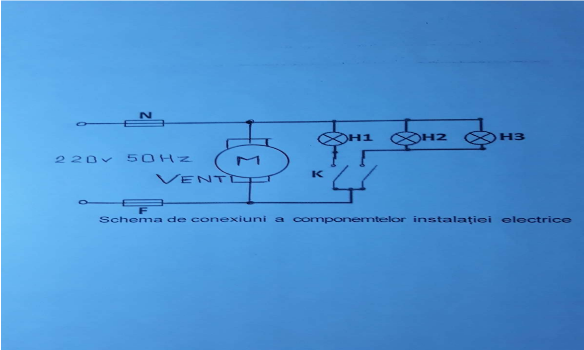
Schema de conexiuni a componentelor dispozitivului antibacterian
